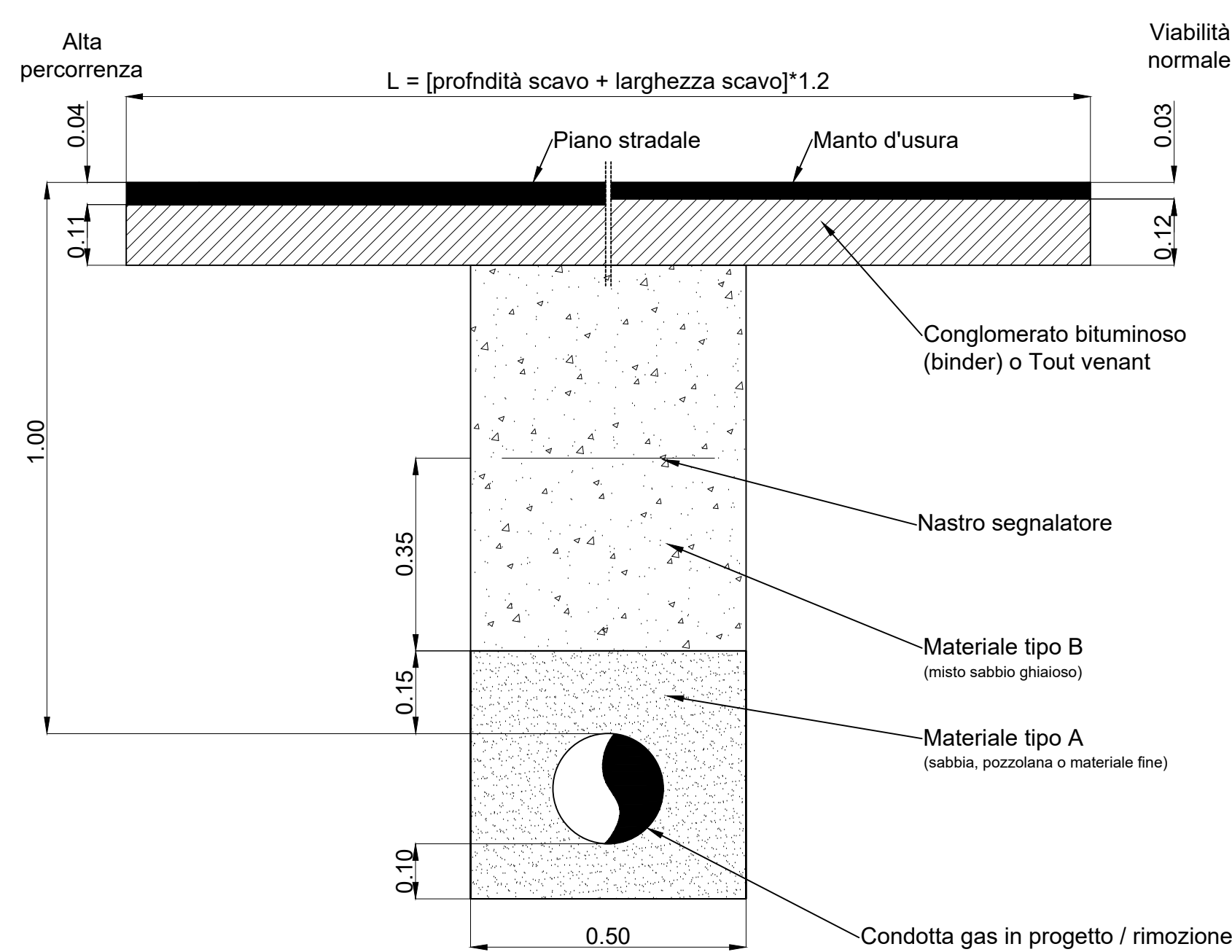
Sezione tipo percorrenza/attraversamento marciapiede strada comunale asfaltata Condotta gas in progetto Pe De 225 - De 180 Condotta gas in rimozione GH DN 150 GH DN 200 - Acc DN 150 - De 180
