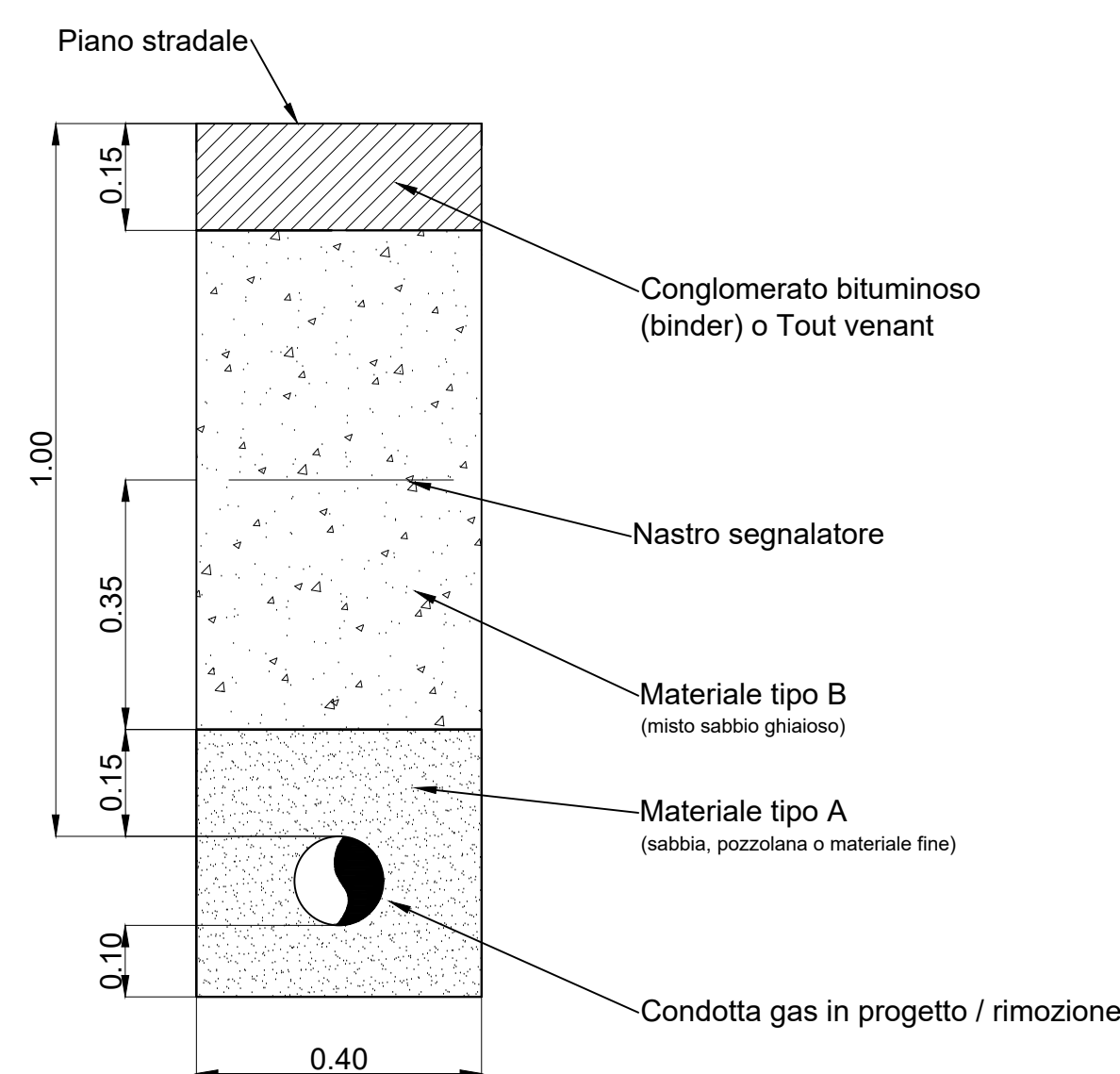
Sezione tipo percorrenza/attraversamento strada privata asfaltata Condotta gas in progetto Pe De 125 Condotta gas in dismissione GH DN 80
