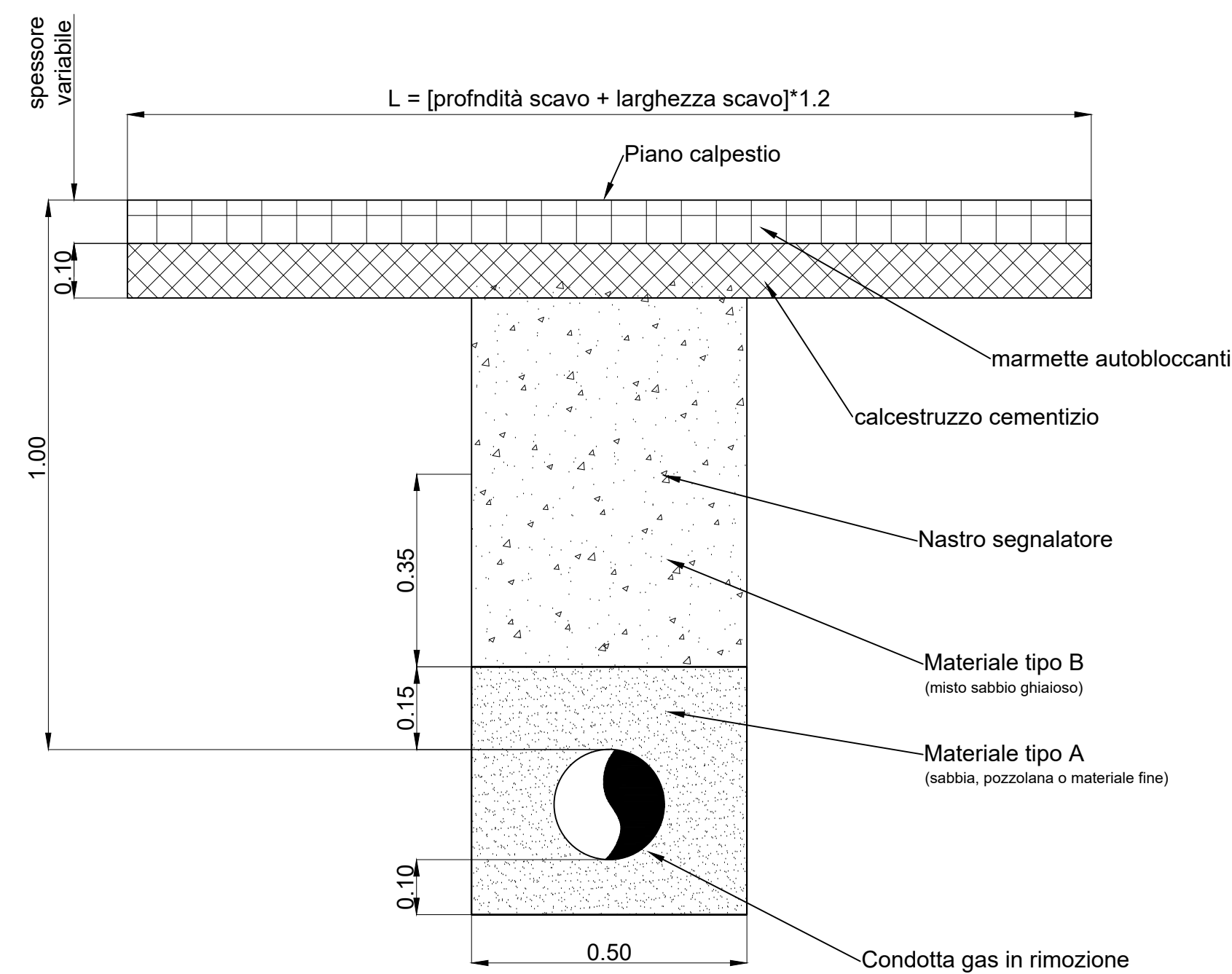
Sezione tipo pavimentazione autobloccanti Condotta gas in progetto Pe De 180 Dismissione GH DN 150
