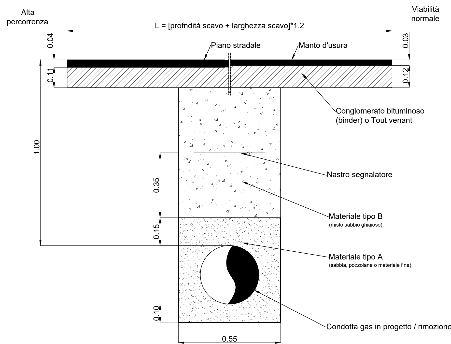
Sezione tipo percorrenza/attraversamento marciapiede strada comunale asfaltata Condotta gas in progetto Pe De 315 Condotta gas in rimozione Acc/GH DN 300/250
