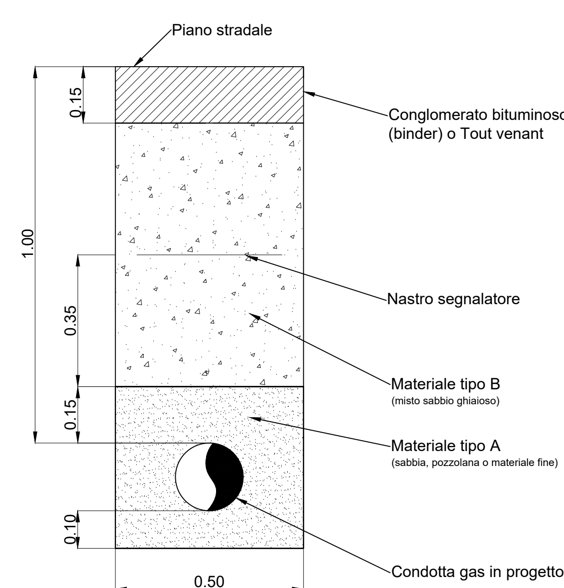
Sezione tipo percorrenza/attraversamento strada privata asfaltata Condotta gas in progetto Pe De 180 Condotta gas in dismissione GH DN 150
