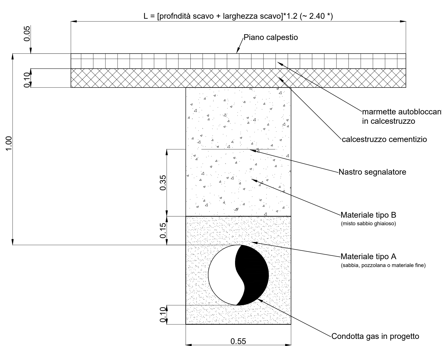
Sezione tipo pavimentazione autobloccanti Condotta gas in progetto Pe De 315 Condotta gas in rimozione ACC/GH DN 250
