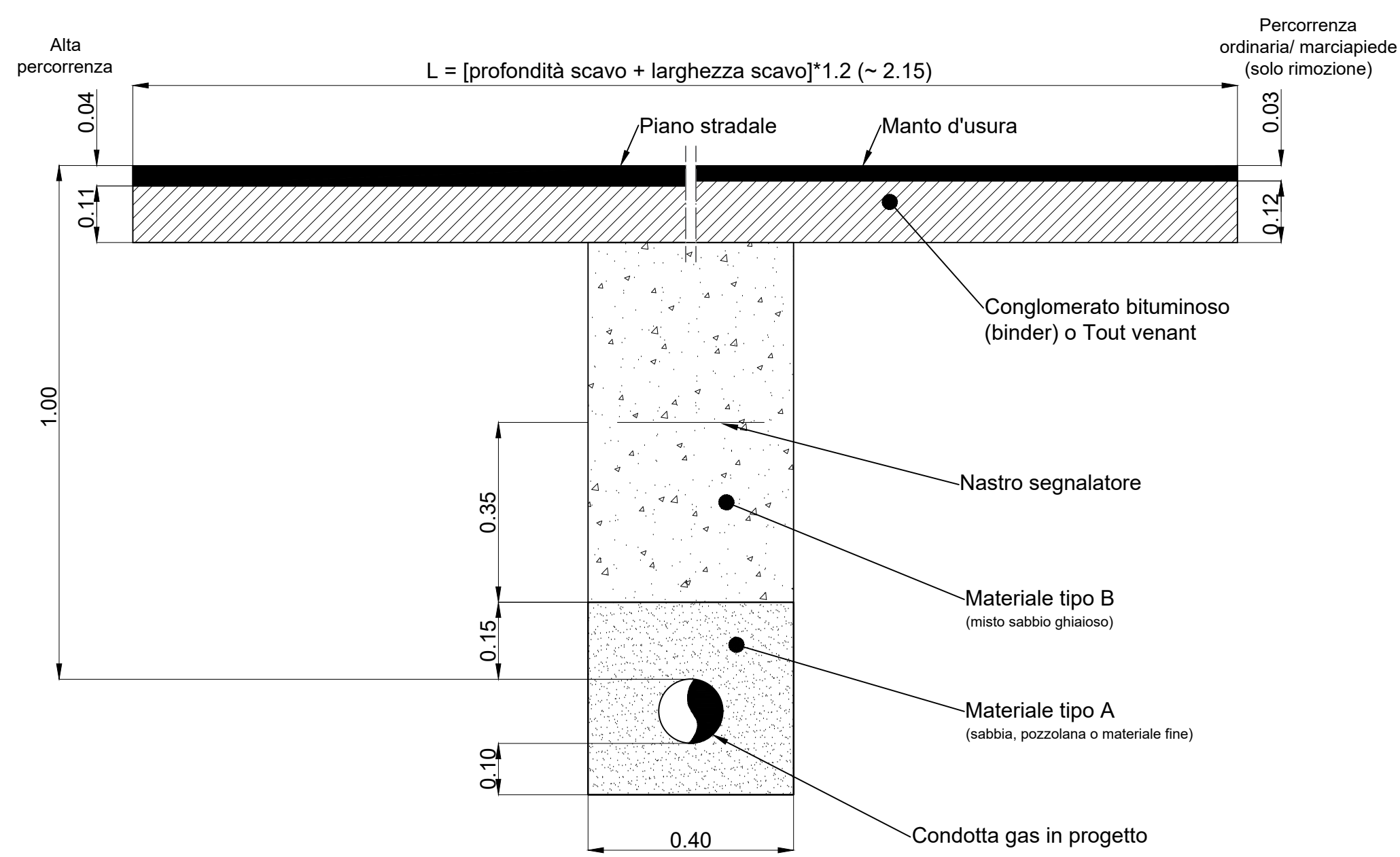
Sezione tipo percorrenza/attraversamento marciapiede strada comunale asfaltata Condotta gas in progetto/rimozione Pe De 125
